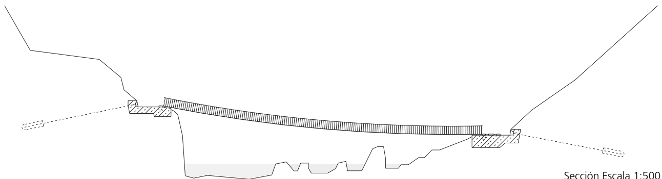
Sección Escala 1:500
